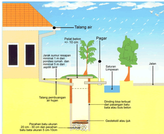
Gambar 2: Sumur Resapan Air
